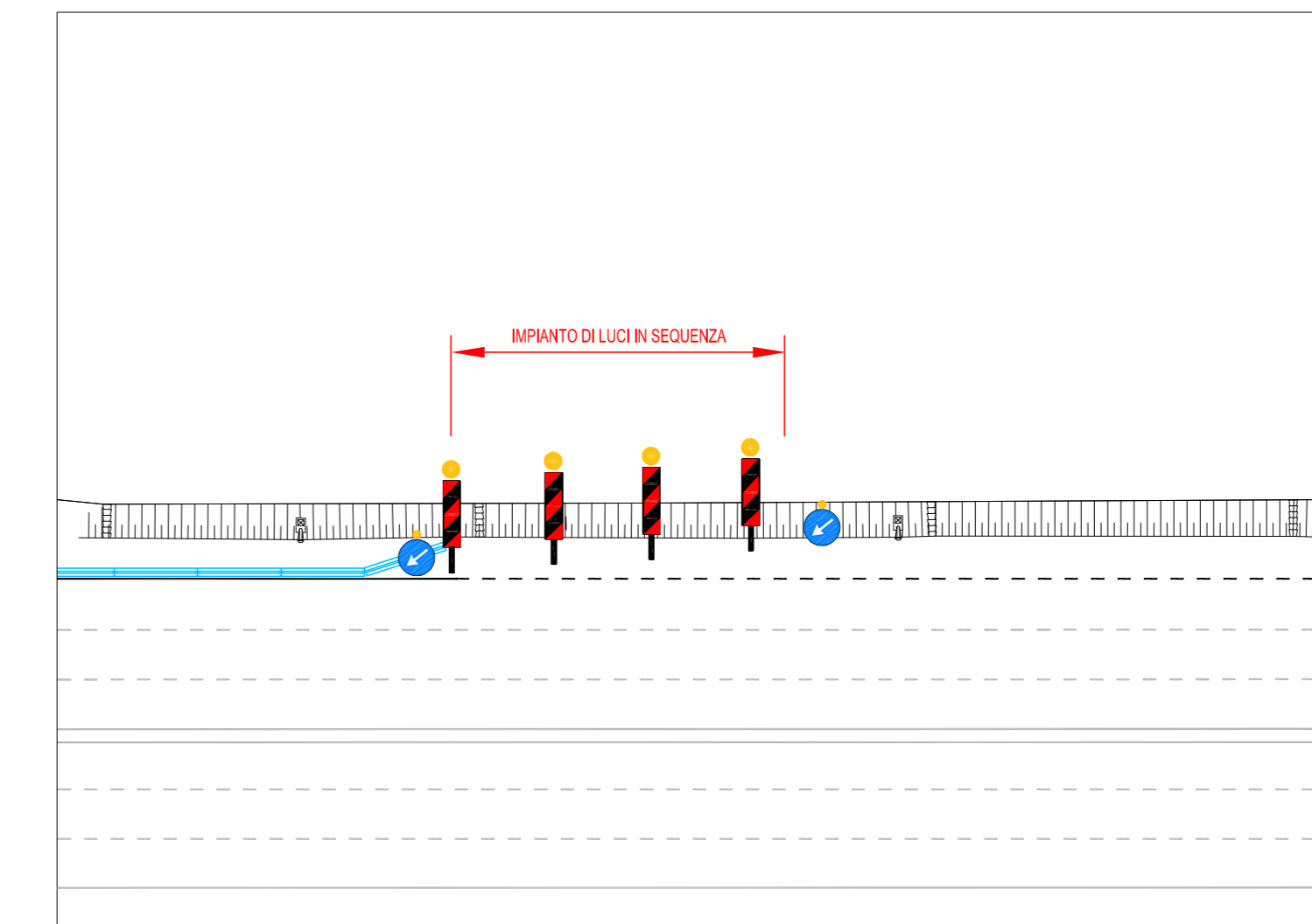
PARTICOLARE POSA LUCI SEQUENZIALI
